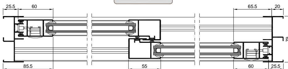
Sección 2 - 2
